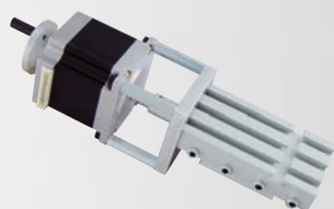
Салазки поперечной подачи
